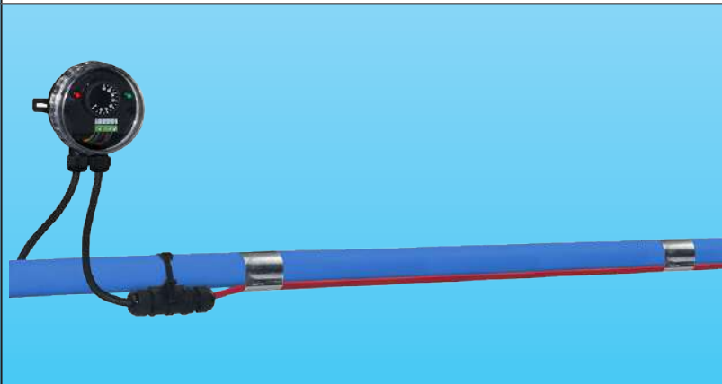
在一根伴热电缆的组装示例，带 Y24 接线盒，用于 PVC 管道的防冻保护
